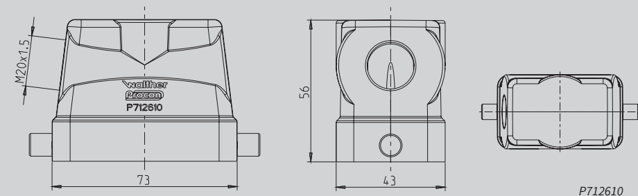
Tüllengehäuse Alu Höhe 56 mm mit Längsverriegelungsbügel Kabeleinführung seitlich
