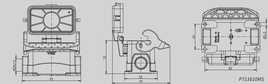
Socket housing Alu Höhe 53 mm mit Längsverriegelungsbügel mit Kunststoff-Klappdeckel
