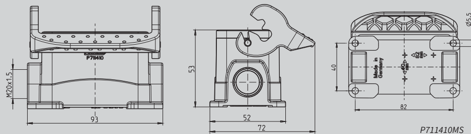
Socket housing Alu Höhe 53 mm mit Längsverriegelungsbügel
