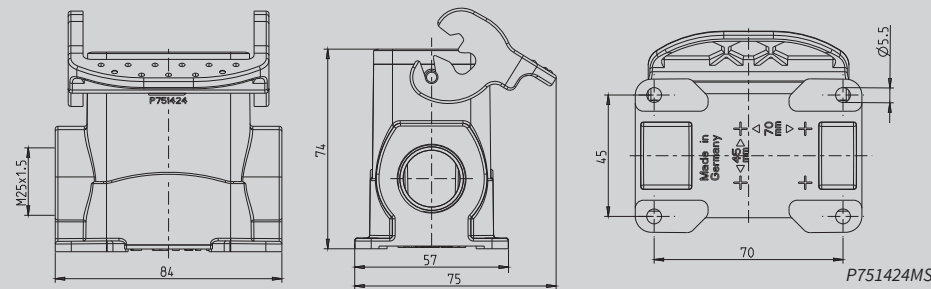
Socketgehäuse Alu Höhe 74 mm mit Längsverriegelungsbügel
