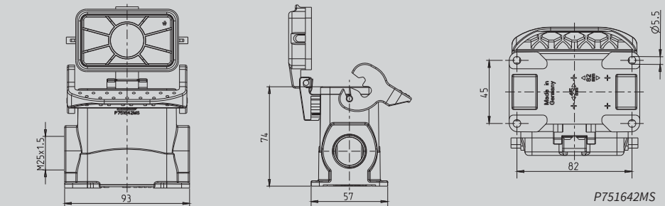
Socket housing Alu Höhe 74 mm mit Längsverriegelungsbügel mit Kunststoff-Klappdeckel
