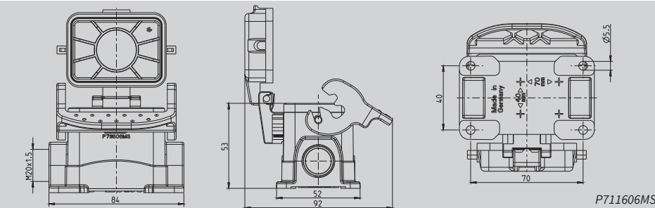
Socketgehäuse Alu Höhe 53 mm mit Längsverriegelungsbügel mit Kunststoff-Klappdeckel
