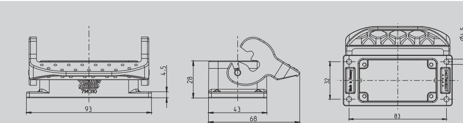
Anbaugeschäuse Alu Höhe 28 mm mit Längsverriegelungsbügel
