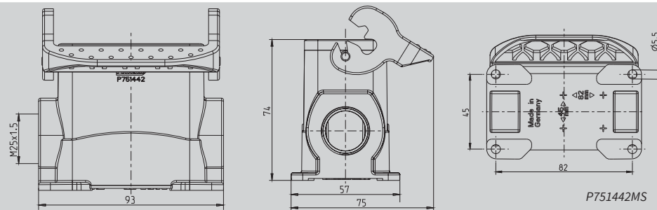
Socket housing Alu Höhe 74 mm mit Längsverriegelungsbügel
