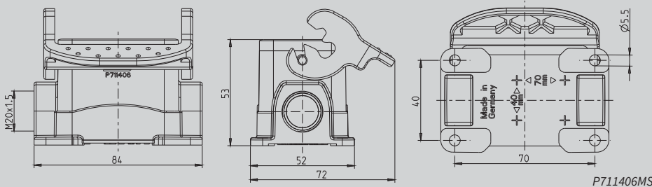
Socketgehäuse Alu Höhe 53 mm mit Längsverriegelungsbügel
