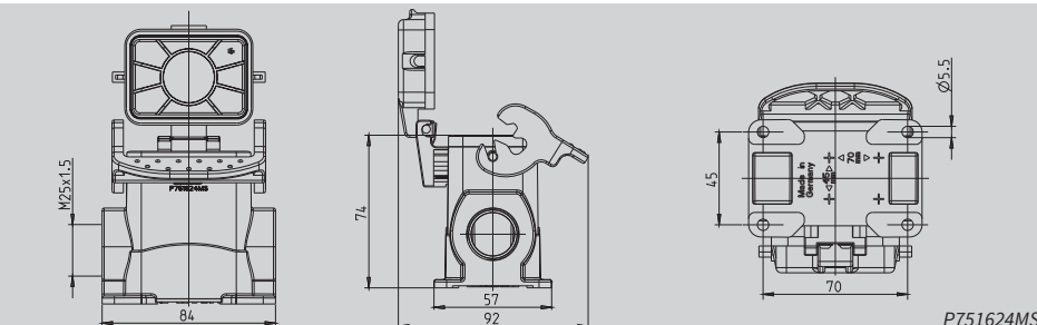
Socketgehäuse Alu Höhe 74 mm mit Längsverriegelungsbügel mit Kunststoff-Klappdeckel
