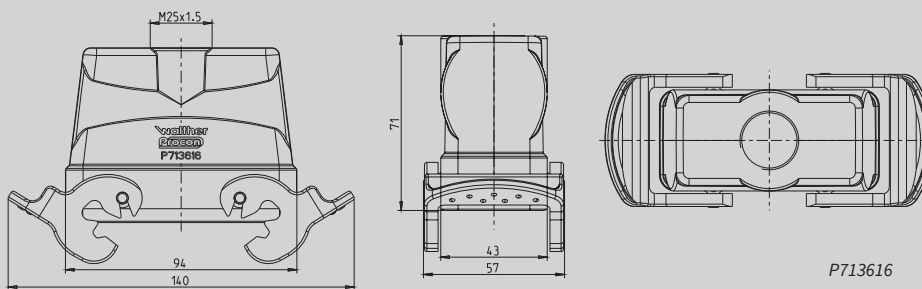
Kupplungsgehäuse Alu Höhe 71 mm mit Querverriegelungsbügeln Kabeleinführung gerade
