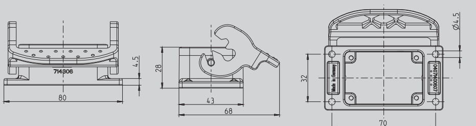
Anbaugehäuse Alu Höhe 28 mm mit Längsverriegelungsbügel
