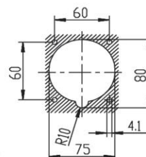
Einbauöffnung
