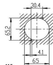
Einbauöffnung
