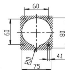
Einbauöffnung
