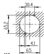
Einbauöffnung
