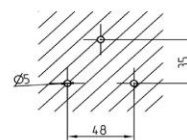
Bohrbild a)
